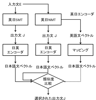
図 4: 自動的なリスコアリングの構成
