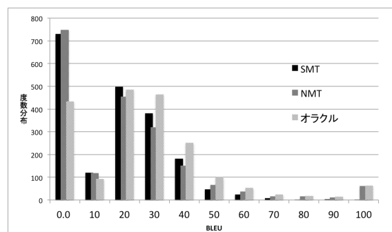
図 5: NMT と SMT のセンテンス BLEU の分布図
