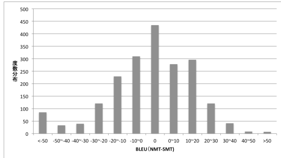
図 6: センテンス BLEU の差分の分布図
