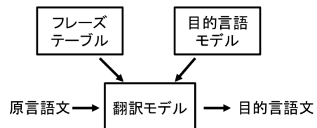
図 1: SMT のブロック図
