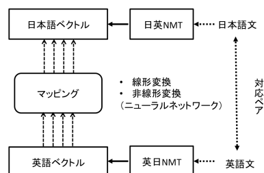
図 3: 文ベクトル間のマッピングの構成
