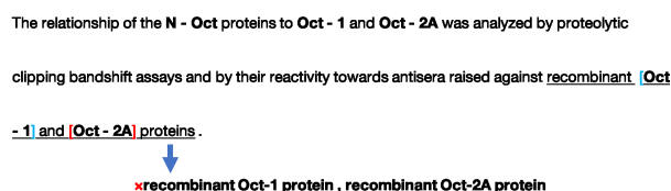
図 2 BioBERT におけるエラー例
