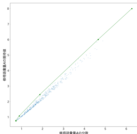
図2 各テキストの修得語彙量分布の期待値と分散。
