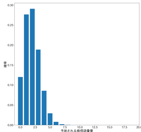
図 1 予測される修得語彙量の分布の例.
