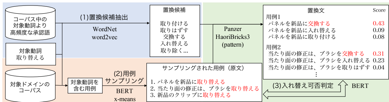
図1 制限語彙の自動構築の流れ（動詞「取り替える」と承認語「交換する」が入れ替え可能か判定する例を示す。）
