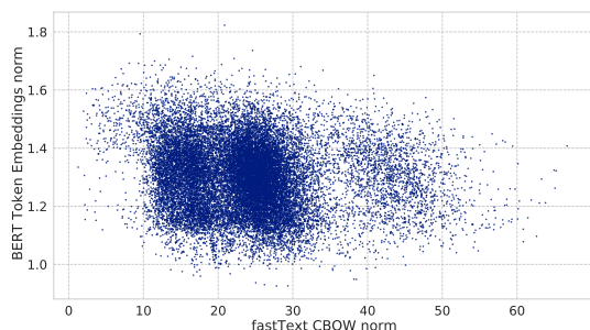
図3 BERT Token Embeddings と fastText CBOW で共通する単語のノルムの関係。相関係数は-0.142。
