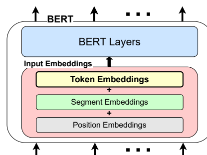
図 1 BERT の構造。BERT Layers は BERT の Input Embeddings 以外の層を表している。
