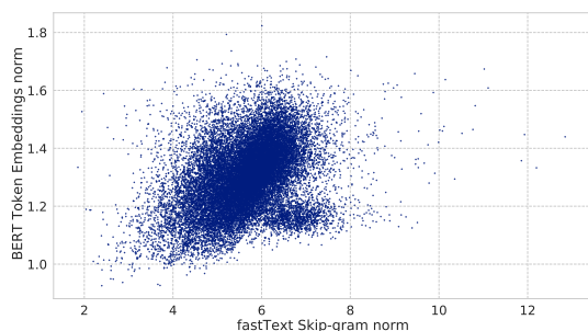
図2 BERT Token Embeddings と fastText Skip-gram で共通する単語のノルムの関係。相関係数は0.355。
