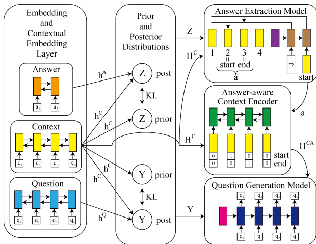
図 1 提案モデルの全体像. 各構成要素の入力と出力が矢印とともに示されている.
